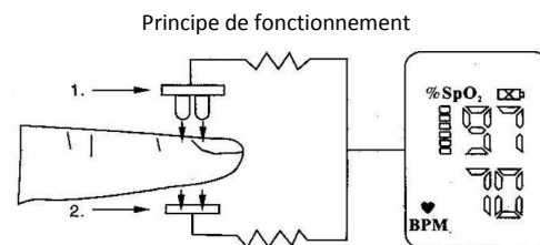
Principe de fonctionnement 1 - Emetteurs Luminescence et infrarouge 2 - Récepteurs Luminescence et infrarouge
